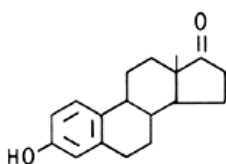
Estrone (E 1 )
