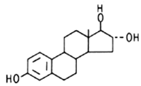
Estriol (E 3 )
