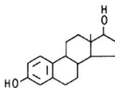
Estradiol -17β(E 2 )
