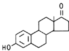
Estrone (E 1 )
