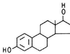
Estradiol -17β(E 2 )
