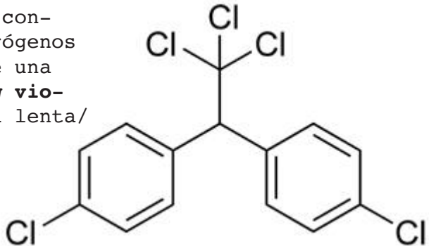
DDT MOLECULE
