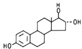
Estriol (E 3 )
